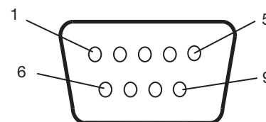
D-SUB 9-pin
